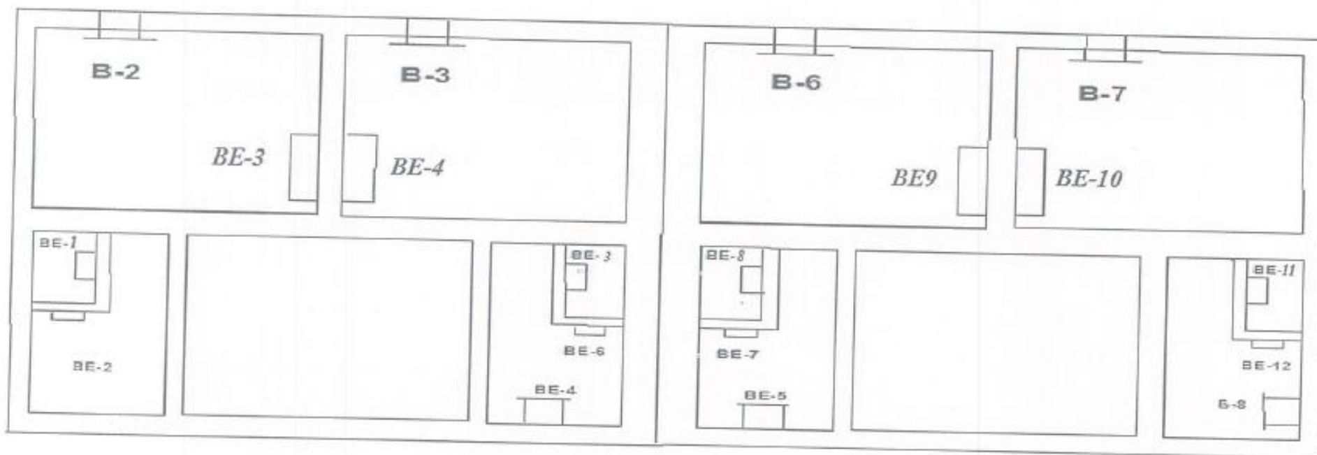
Схема расположения вентиляционных систем в санитарно-бытовом блоке ПРЦЭО ПУ «Жетыбаймунайгаз»
